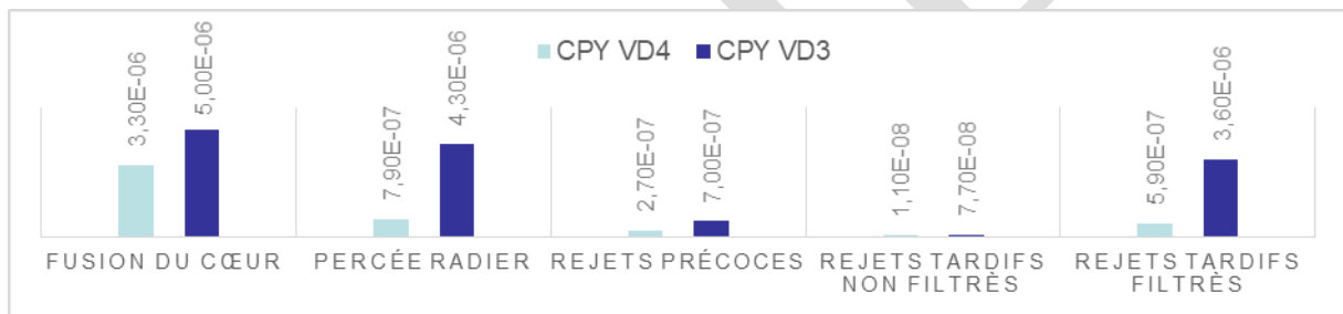
Figure 1 : Risque de rejets dans l'environnement à la suite d'un événement interne (évaluations d'EDF)
