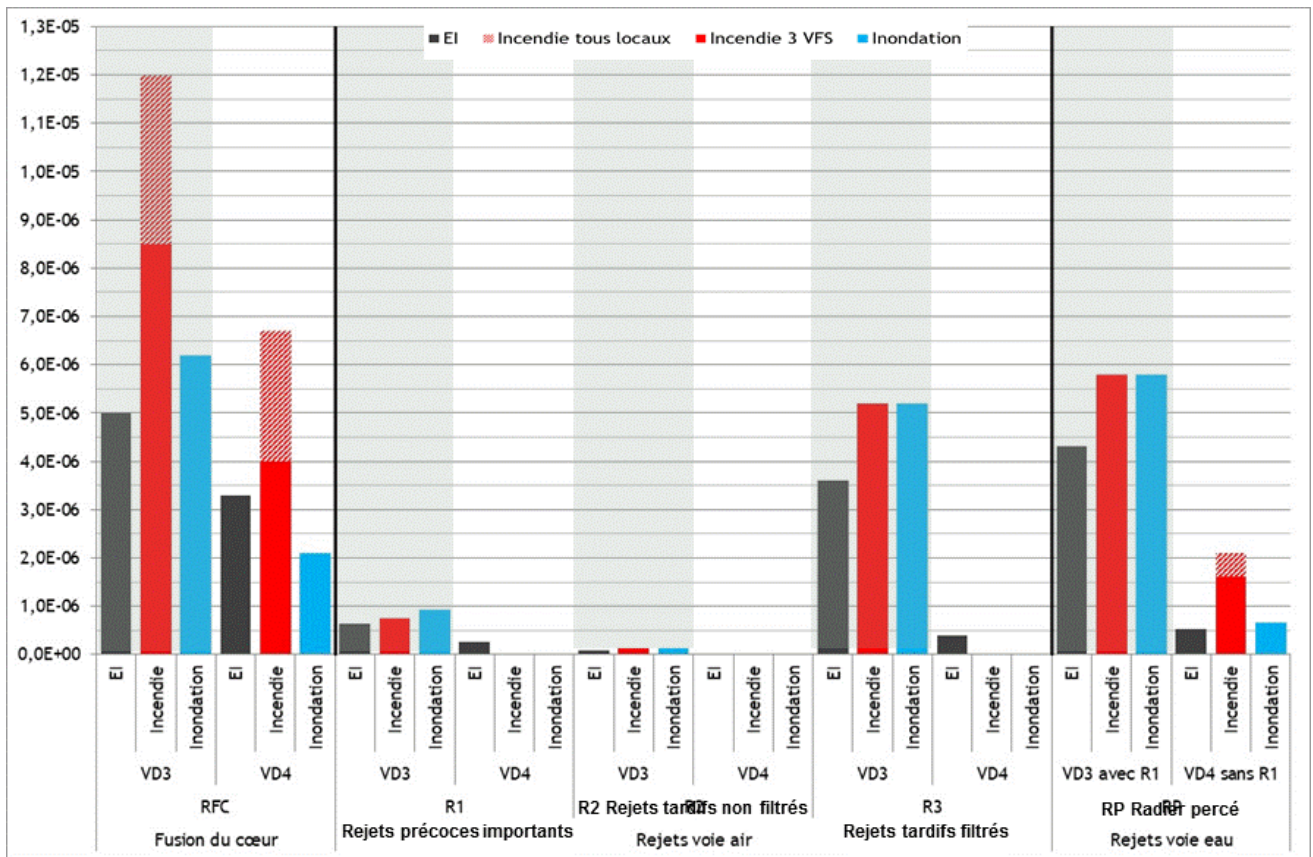
Figure 2 : Risque de rejets dans l'environnement en cas d'agression d'origine interne (évaluations d'EDF)
